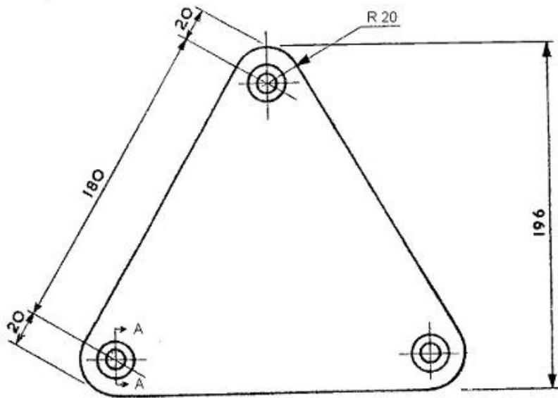
Τρίποδο ηλεκτρόδιο
